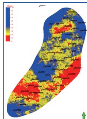
0m slice
