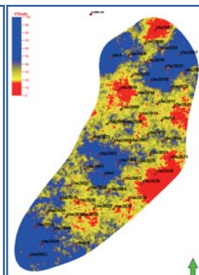
6.0m slice
